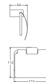
B91009 Держатель для полотенец
