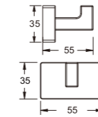
B90304 Держатель для полотенец
