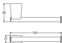
B91103 Держатель для ТБ
