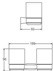
B91103-2 Держатель для ТБ
