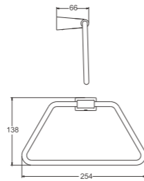
B91512 Держатель для полотенец
