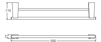
B91415-4 Планка с крючками (4)
