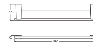
B91215-4 Планка с крючками (4)
