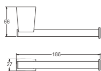
B91303 Держатель для ТБ
