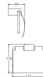
B90909 Держатель для полотенец
