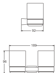
B91303-2 Держатель для ТБ
