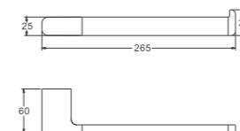
B91001 Держатель для полотенец
