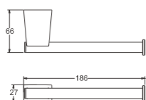
B91203 Держатель для ТБ
