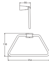
B91412 Держатель для полотенец
