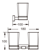
B90203 Держатель для ТБ
