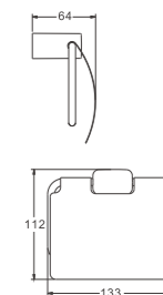
B90809 Держатель для полотенец
