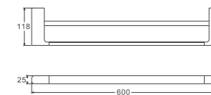
B90924 Полка для полотенец
