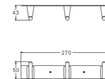
B91115-5 Планка с крючками (5)
