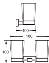
B90303 Держатель для ТБ
