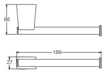
B91403 Держатель для ТБ
