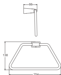
B91212 Держатель для полотенец
