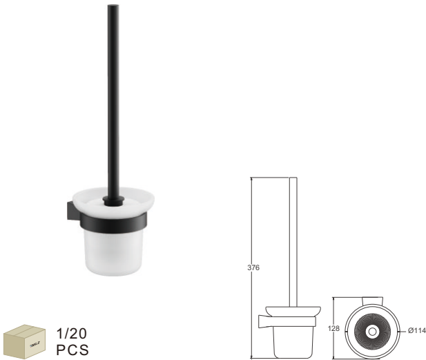
B91410 Ёршик
