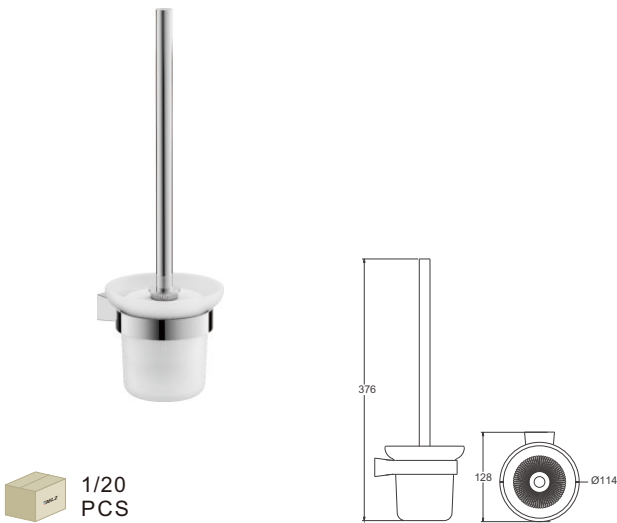
B91110 Ёршик
