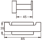
B90302-1 Мыльница
