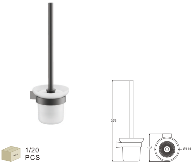
B91210 Ёршик
