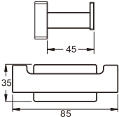
B90402-1 Мыльница
