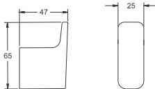
B90727 Дозатор
