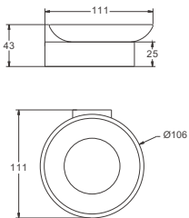
B90708 Стакан
